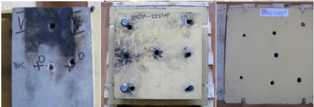
Rys 21 Badania próbek materiałowych pancerzy
